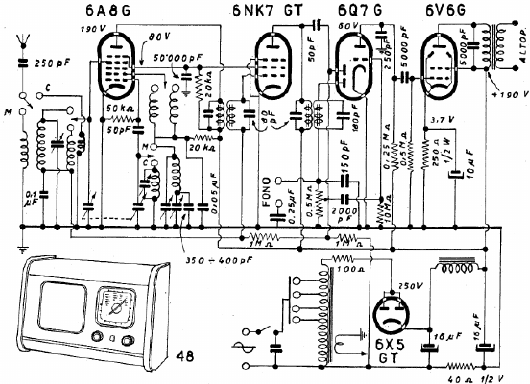
WATT RADIO - Mod. WATT 48 - Gamma medie da 590 a 187 m, gamma corte da 55 a 18 m. Media frequenza 460 kc/s. Sensibilità di potenza 0,4 mV. Potenza d'uscita 3 W. Consumo 35 W.
